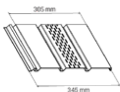
Perforované podbití
