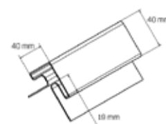
Rohová lišta
